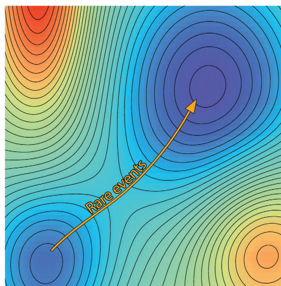
Free energy
